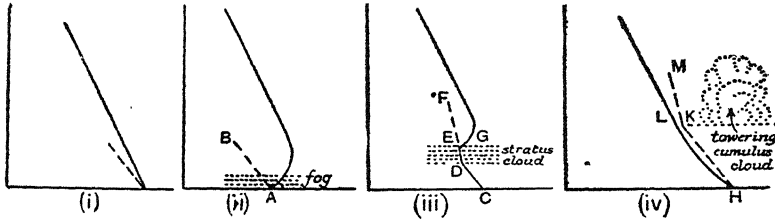
चित्र ४९ (b) जब वायु ठंडे और गर्म सतहों पर चलती है तब स्थायित्व पर प्रभाव
